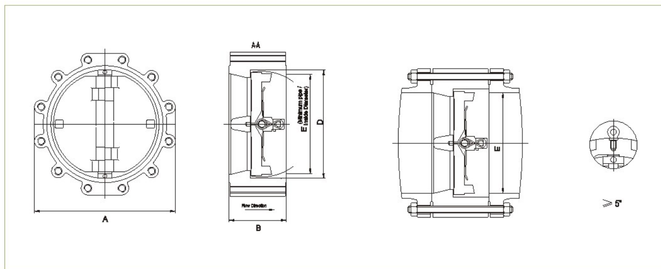
Lug type
